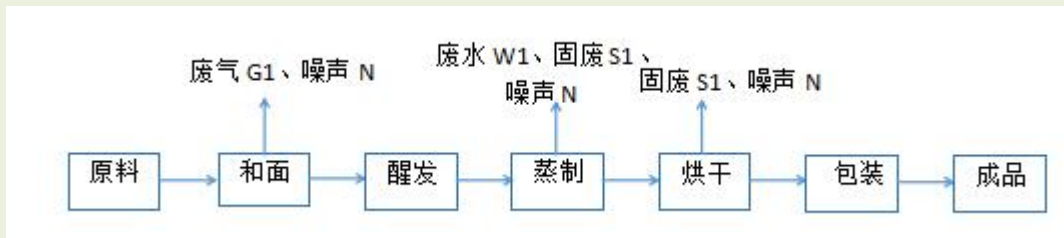
图2 生产工艺流程及产污环节图
